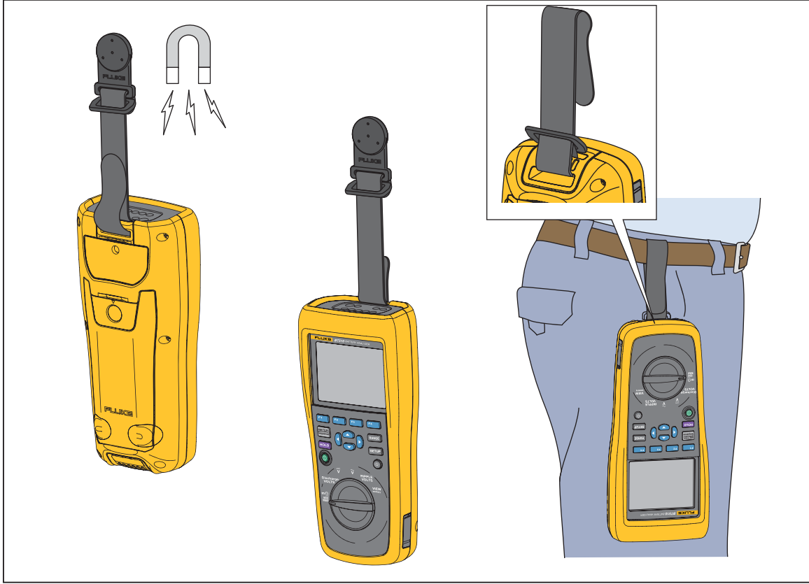
Şekil 2-2. Kemer Askısı
