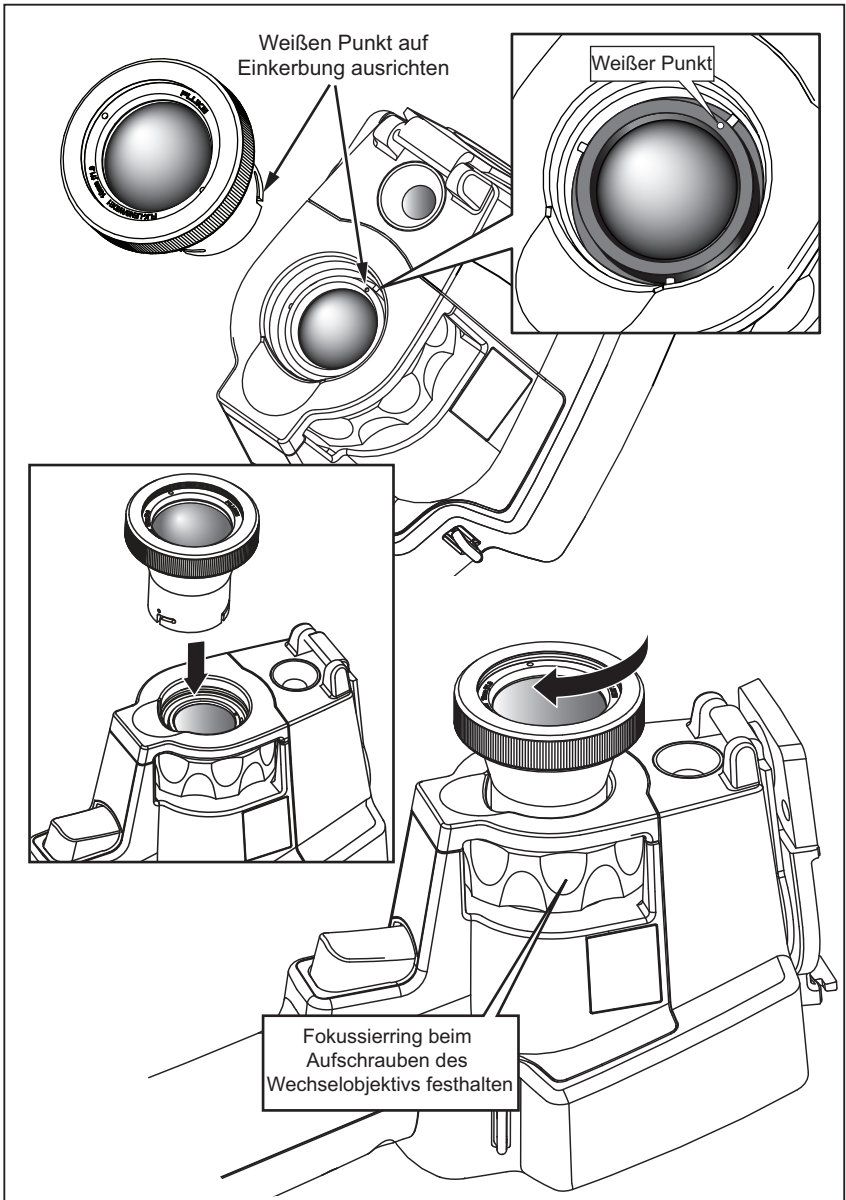
Abbildung 1. Anbringen und Abnehmen der optionalen Objektiv
