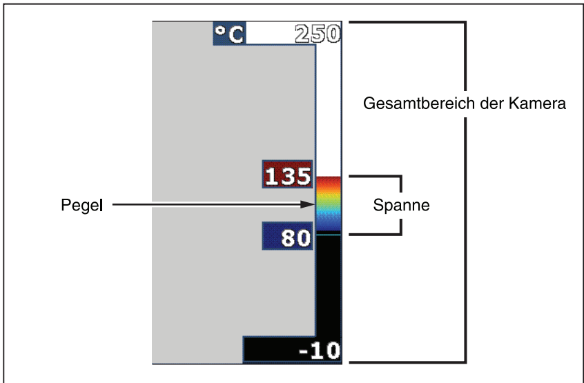
Abbildung 2. Bereichs- und Spanne-Einstellungen
