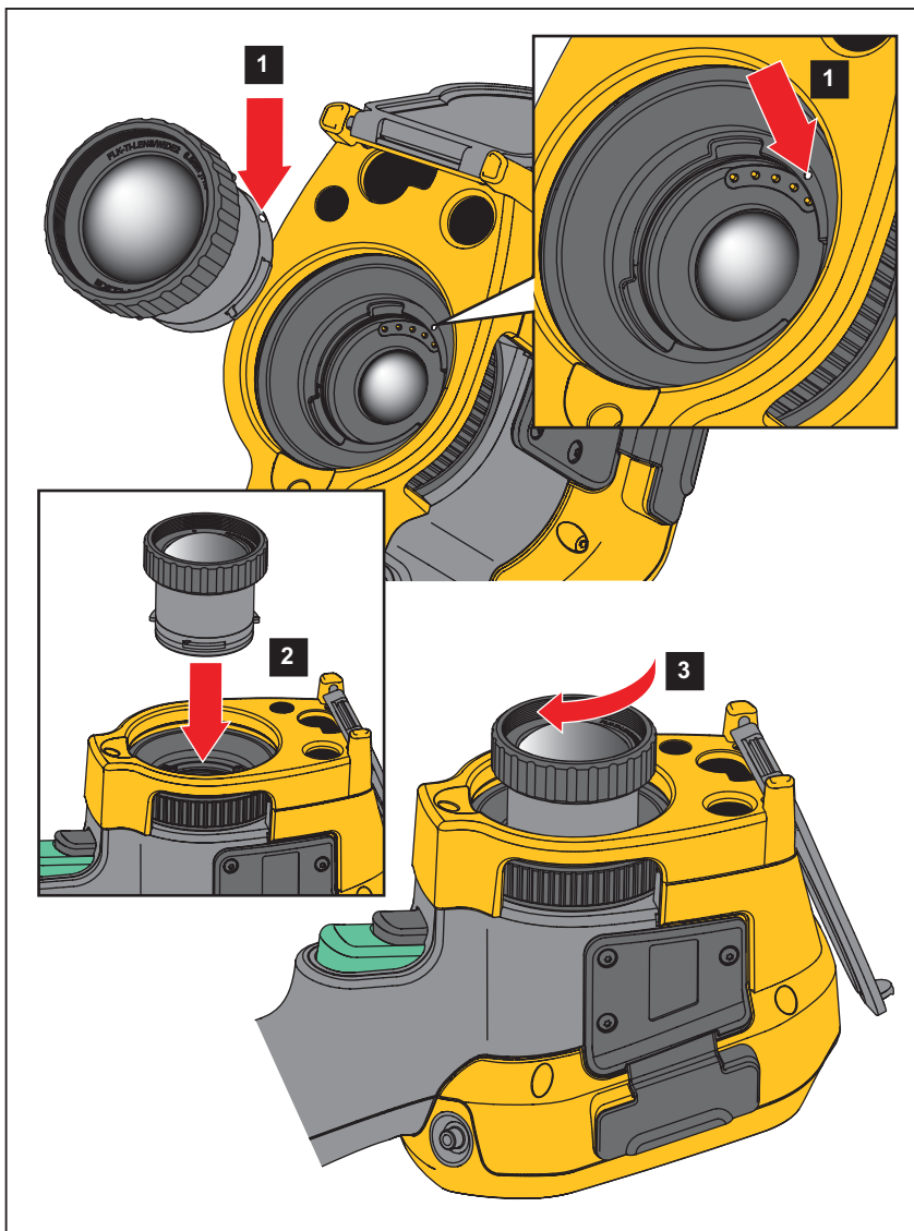
Figura 1. Instalação de lente opcionais
