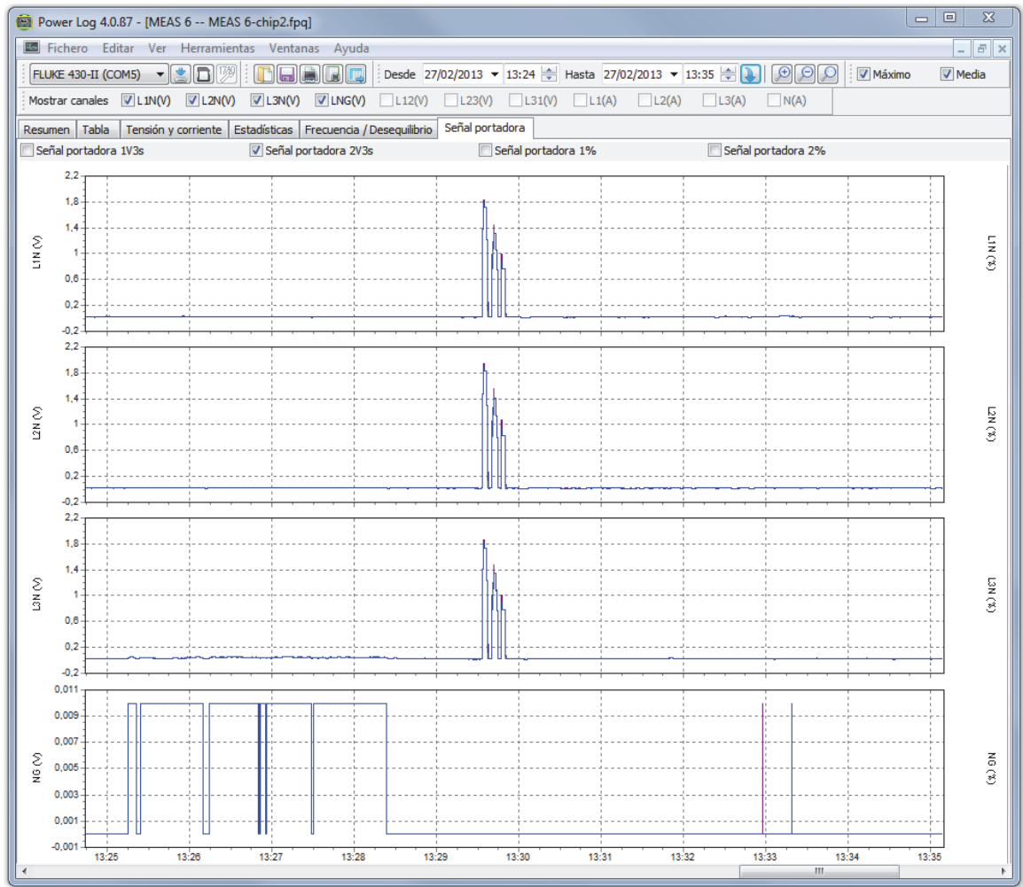
Figura 18. Formas de onda de la señal portadora
