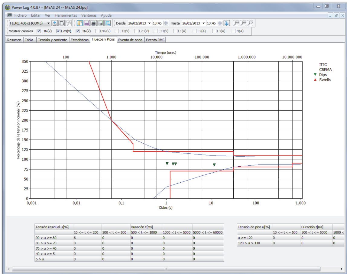
Figura 9. Huecos y picos
