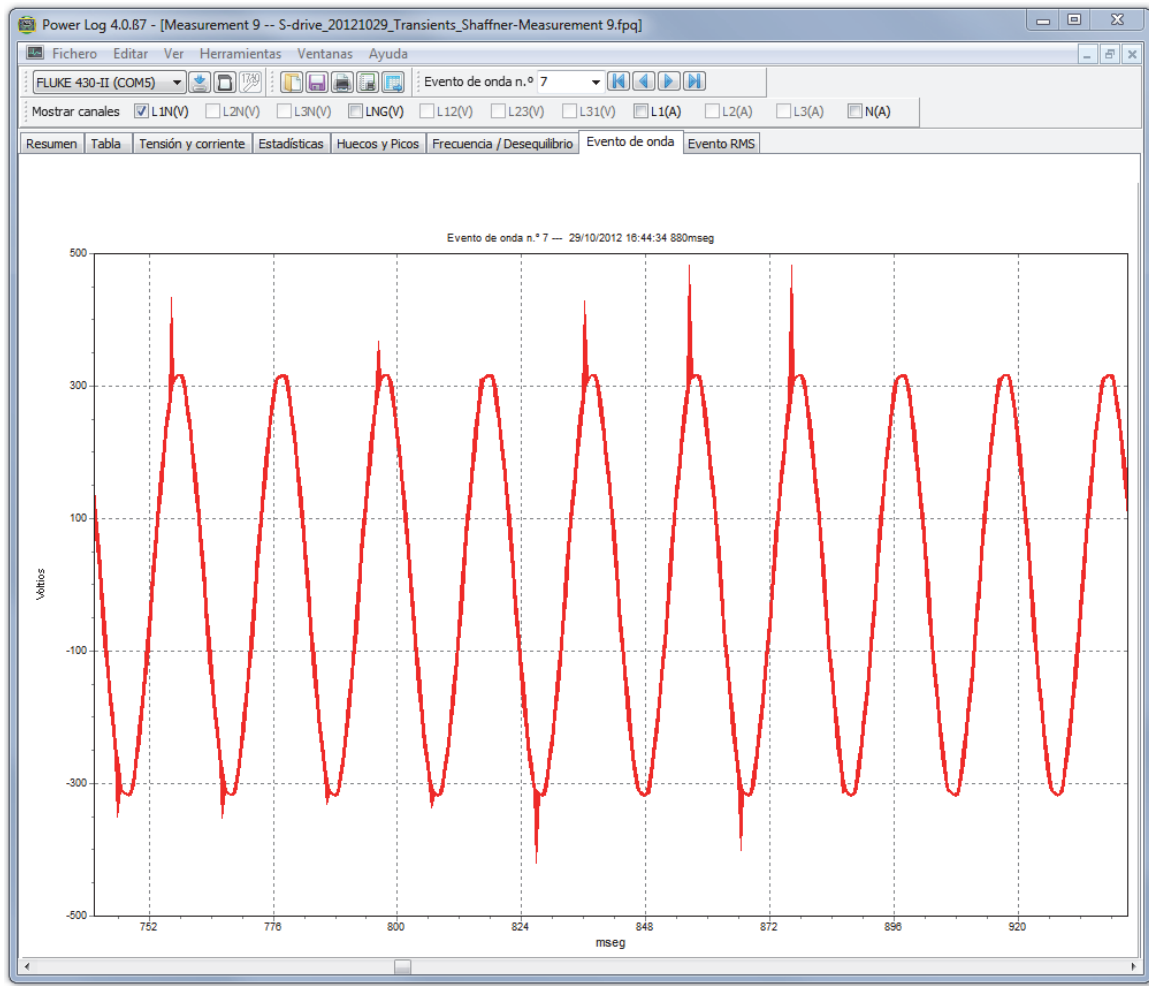
Figura 12. Forma de onda de transitorio
