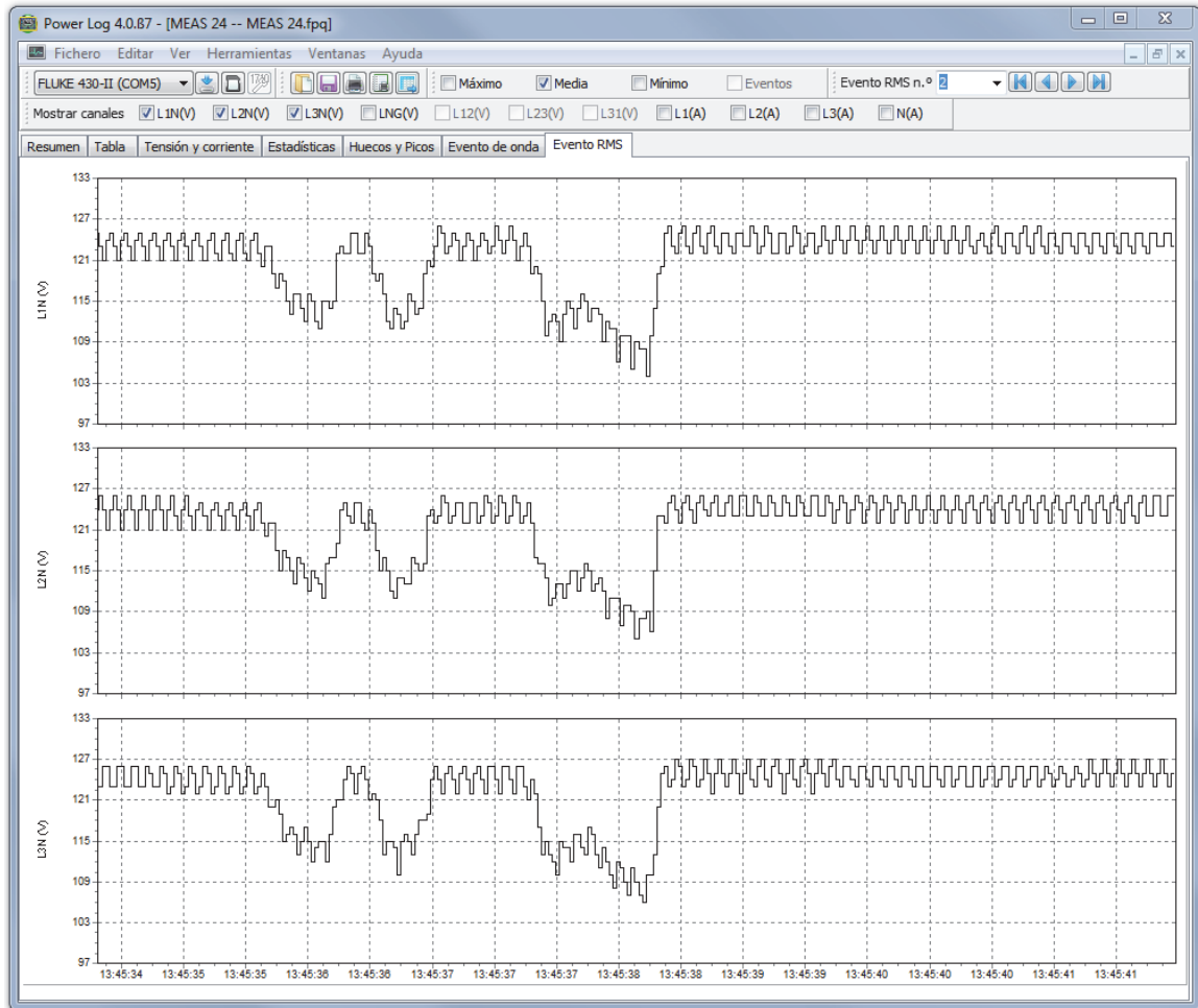
Figura 16. Perfiles de tensión
