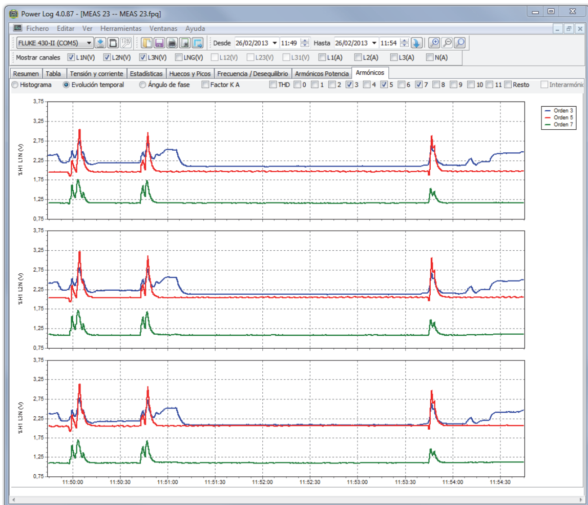
Figura 7. Evolución temporal de armónicos con los canales seleccionados
