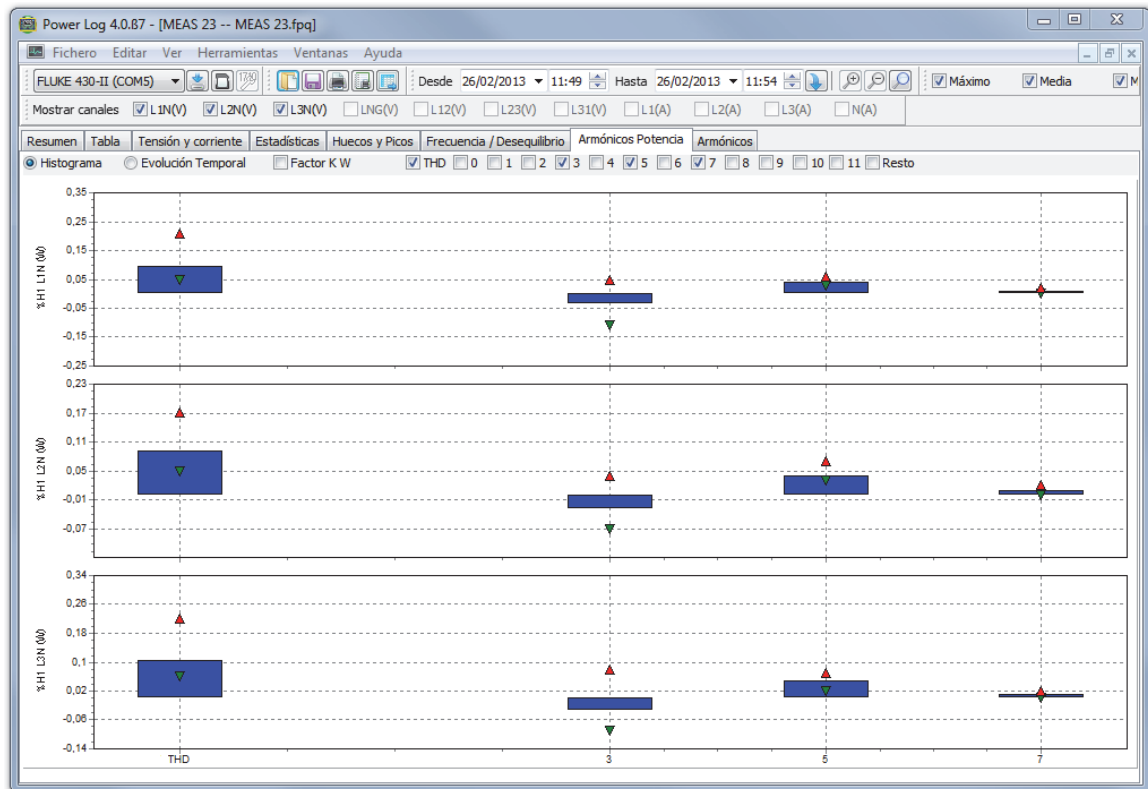
Figura 17. Armónicos de potencia
