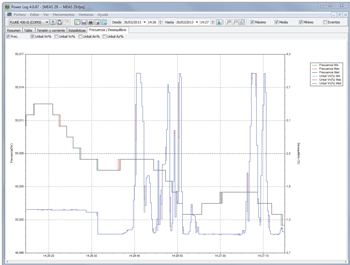
Figura 10. Gráfico de tiempo de Frecuencia/Desequilibrio: Frecuencia
