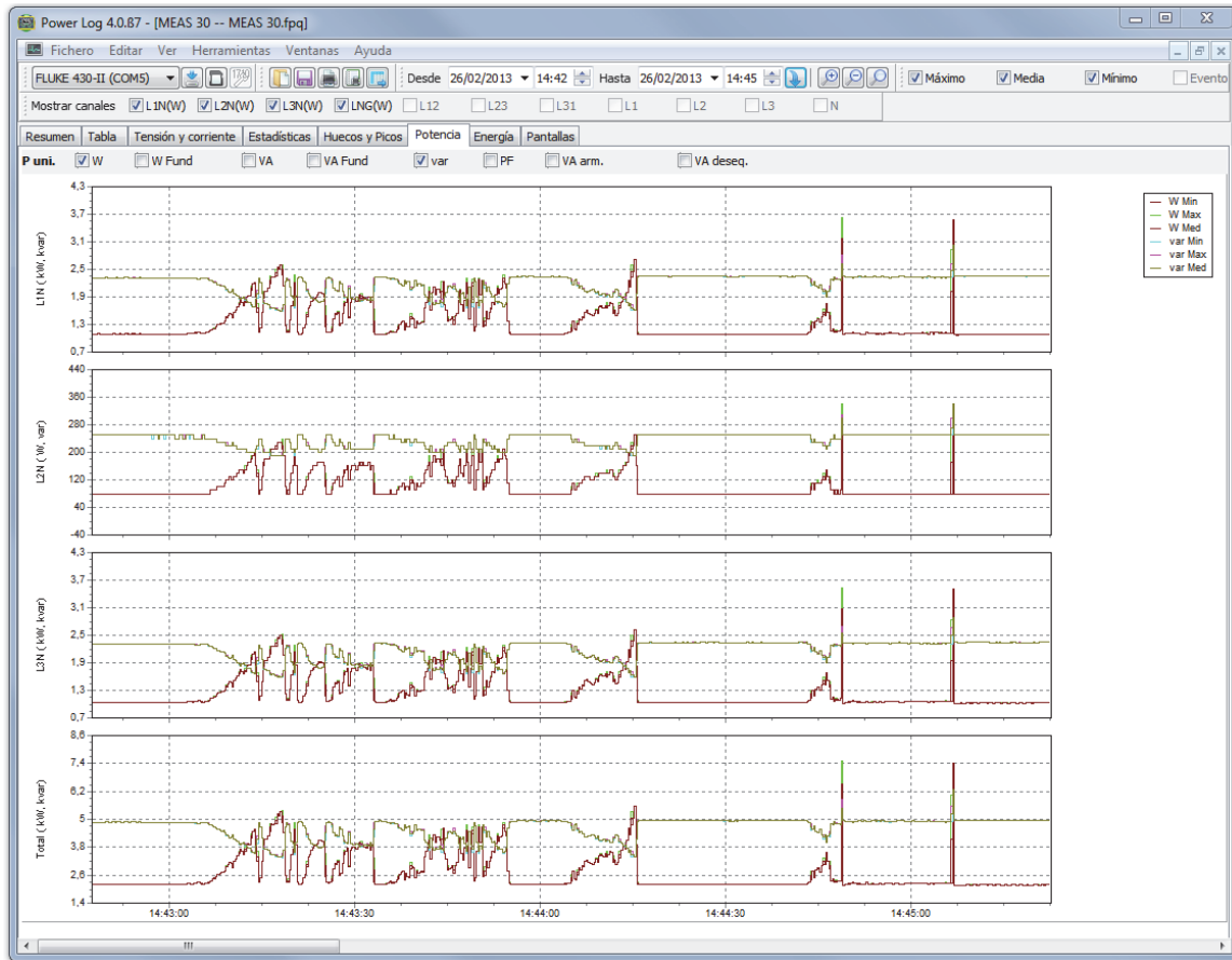
Figura 11. Gráfico de tiempo de potencia con potencia activa y reactiva seleccionada
