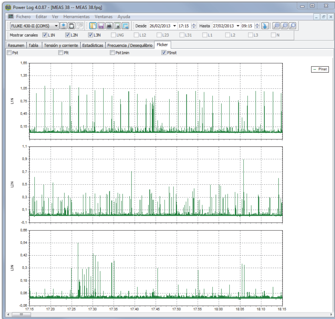
Figura 13. Formas de onda de Flicker
