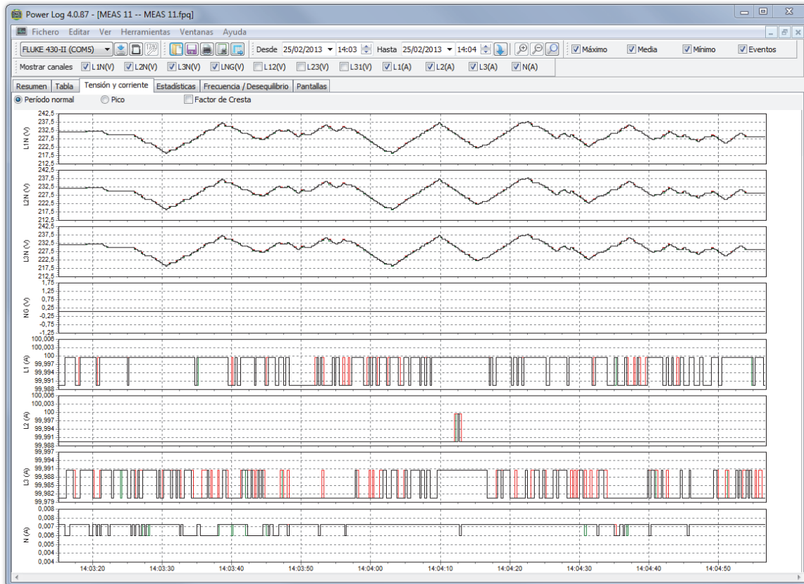
Figura 5. Gráfico de tiempo de tensión y corriente con los canales seleccionados visibles
