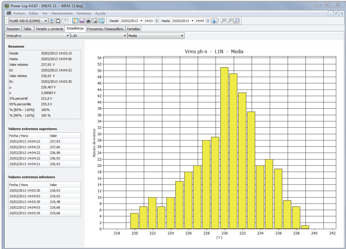
Figura 6. Estadísticas con el canal A seleccionado
