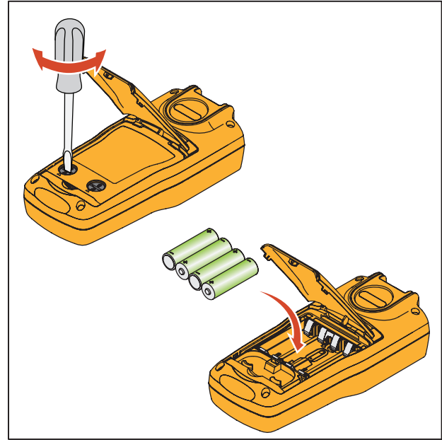
그림 8. 배터리 교체
