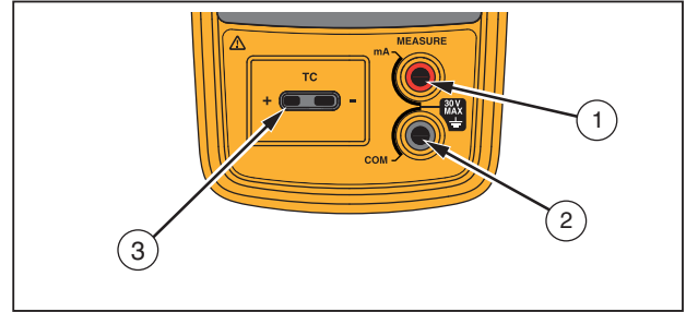
그림 2. 입력/출력 단자와 커넥터
