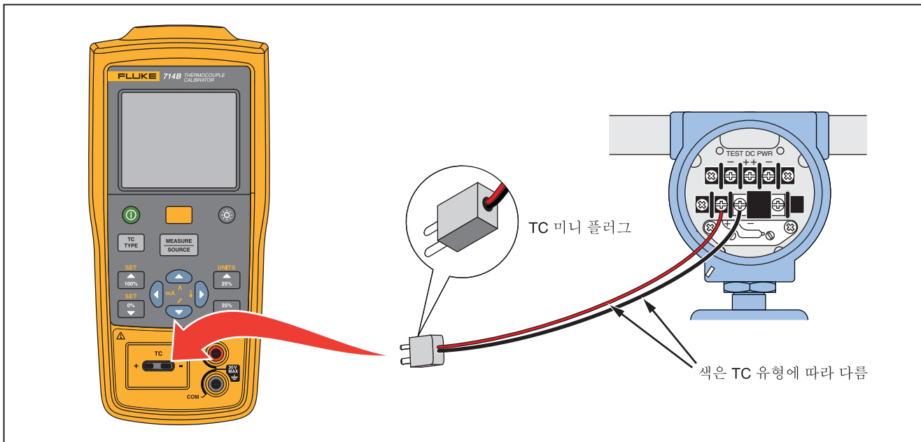
그림 7. 열전쌍 시뮬레이션을 위한 연결
