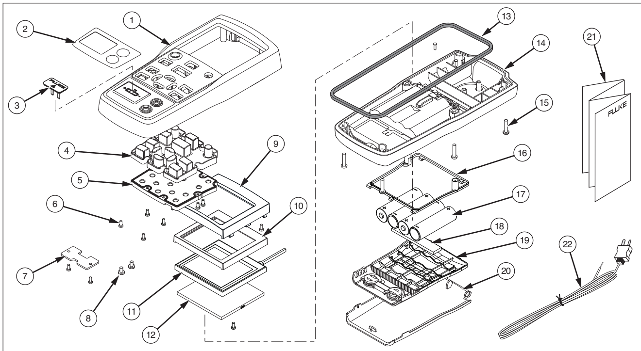
그림 9. 교체 부품
