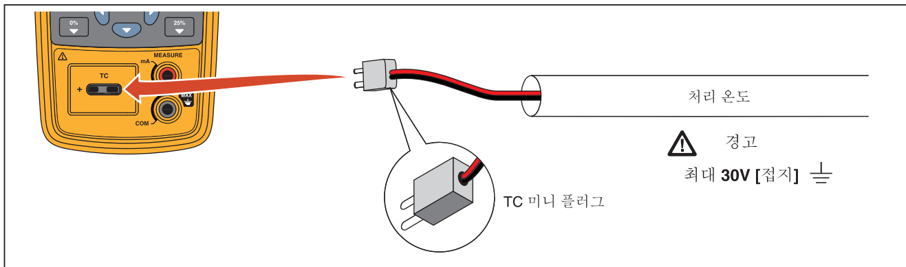
그림 6. 열전쌍으로 온도 측정하기
