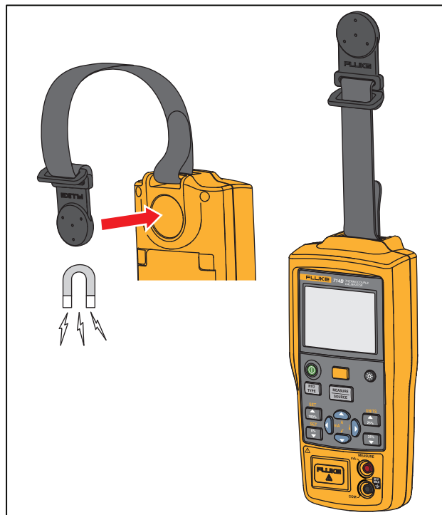
그림 5. 걸이 스트랩으로 자석 장착하기
